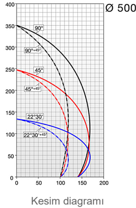
Kesim diagramı
