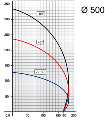
Kesim diagramı
