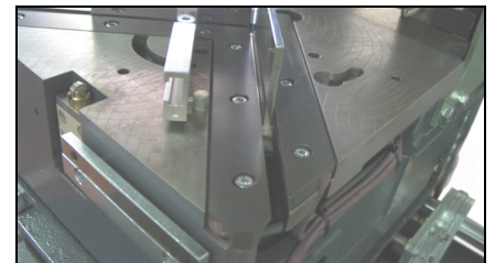
Schweißraupenbegrenzung durch beheizte und einstellbare Messer
