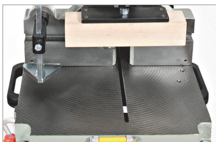
切割区
