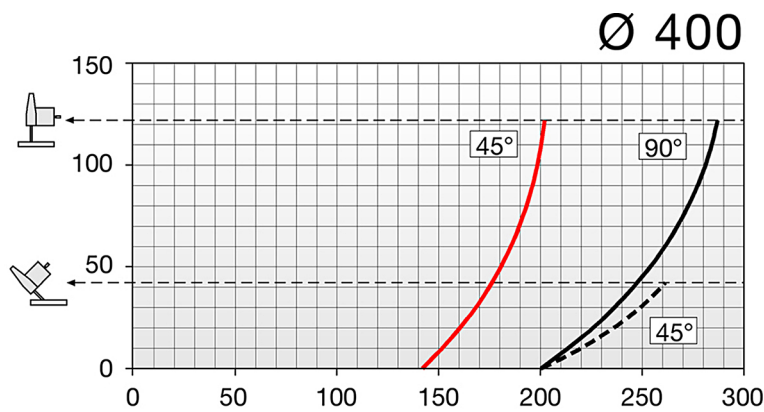
切割曲线图
