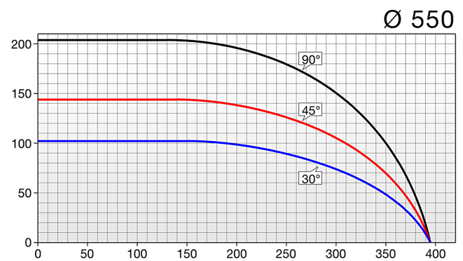
切割曲线图
