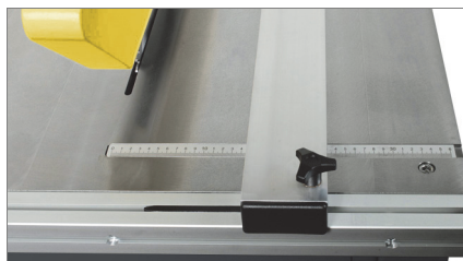
Dettaglio battuta regolabile 01
