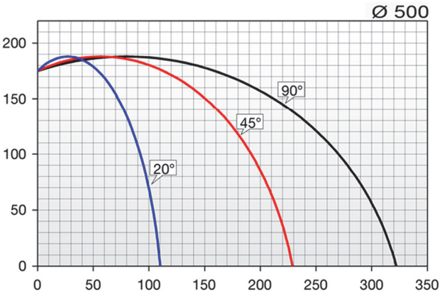
切割曲线图
