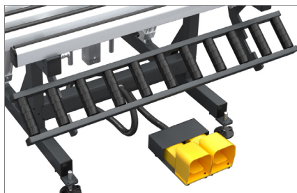
Base de rodillos para desplazamiento de la carpintería 04
