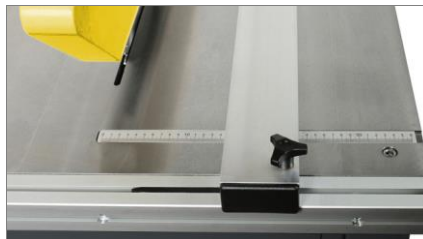
Detailansicht des verstellbaren Werkstückanschlags 01
