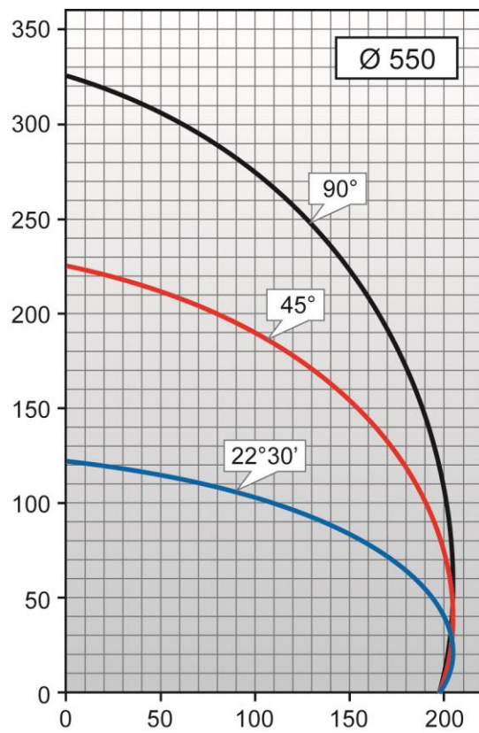
Schnittdiagramm
