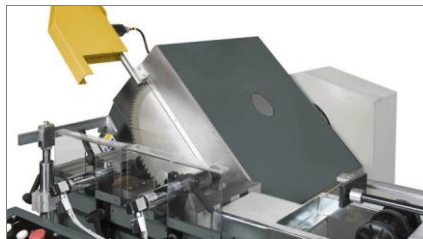
45° / 22°30' Sägeaggregat 01
